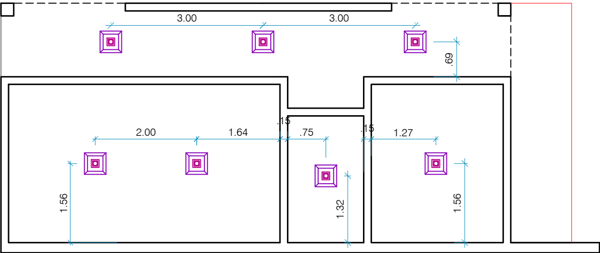
PLANTA BAIXA PONTOS LUMINICOS _____ 1/75
